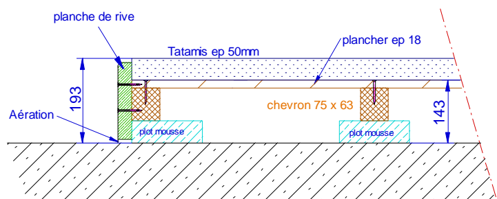
Plancher sur dalle béton
