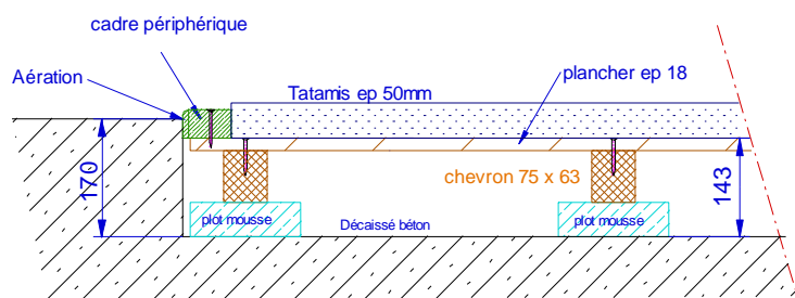
Plancher dans un décaissé béton
