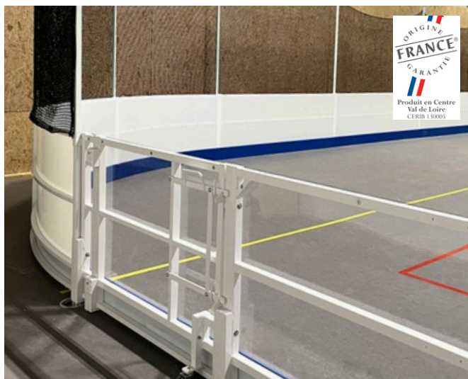
HK2001 RAMBARDE DE RINK HOCKEY / ROLLER HOCKEY EN POLYÉTHYLÈNE HAUTE DENSITÉ (PEHD) ET POLYCARBONATE SUR MESURE
